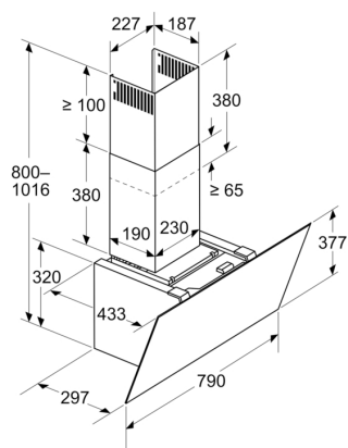
Mått i mm Enheten är i cirkulationsluftläge
