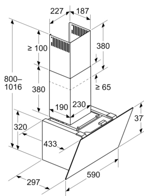
Mått i mm Enheten är i cirkulationsluftläge
