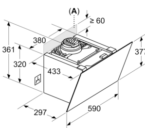
Mått i mm Enheten är i cirkulationsluftläge utan kanal
