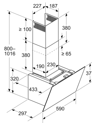
Mått i mm Enheten är i cirkulationsluftläge
