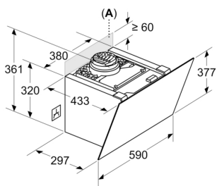
Mått i mm Enheten är i cirkulationsluftläge utan kanal
