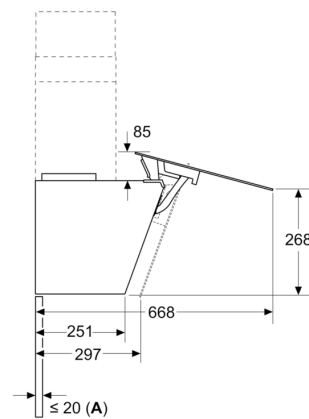
Mått i mm
