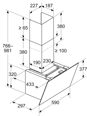
Mått i mm Enheten är i evakueringsläge
